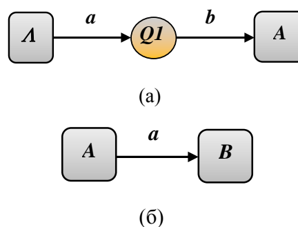
Рис. 6. Базовые фрагменты конечного автомата для распознавания паттернов данных науки, образования и инновационной деятельности
