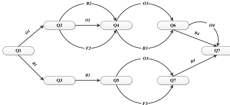
Рис. 7. Конечный автомат для распознавания паттернов данных науки, образования и инновационной деятельности
