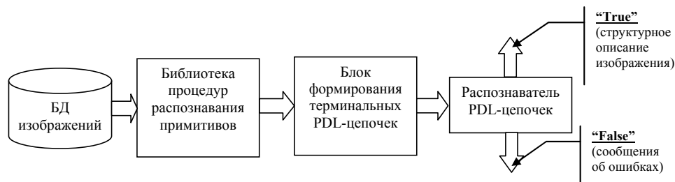
Рис. 1. Общая схема распознавания изображений, специфицированных в языке PDL
