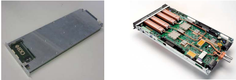
Рис. 6. Слева — плата «СКИФ-Аврора», справа — плата «Aquasar»
