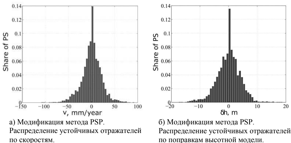
Рис. 3. Распределения скоростей смещения и поправок априорной высотной модели для модификации метода PSP
