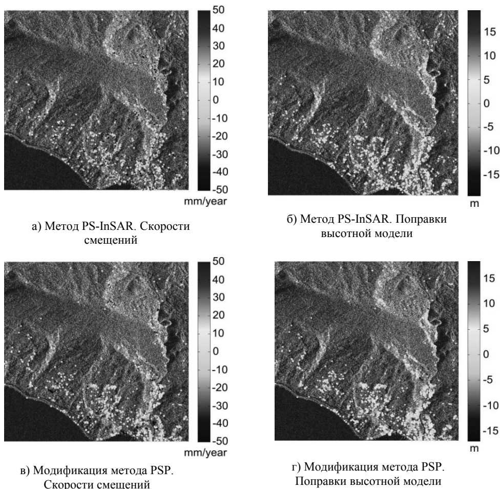
Рис. 2. Сравнение результатов интерферометрической обработки РЛ снимков (скорости смещений и поправки высотной модели) для метода PS-InSAR и модификации метода PSP
