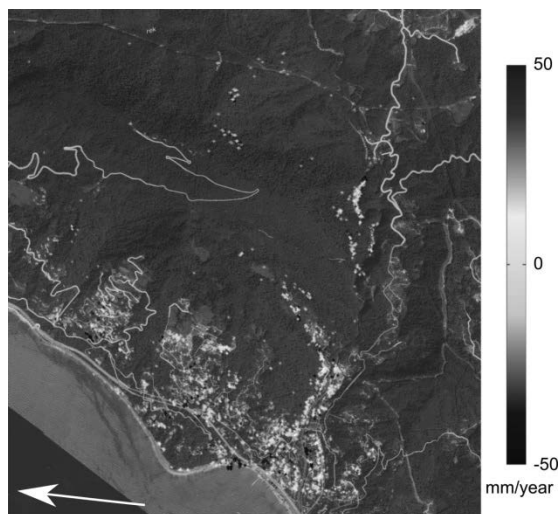
Рис. 4. Карта смещений земной поверхности, полученная при применении предложенной модификации метода PSP (картографические данные: © Google, DigitalGlobe, 2013)
