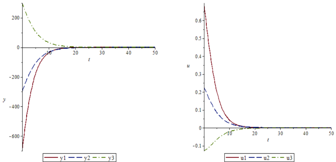
Рис. 1. Графики y(t) и субоптимального управления u(t) без ограничений на управление
