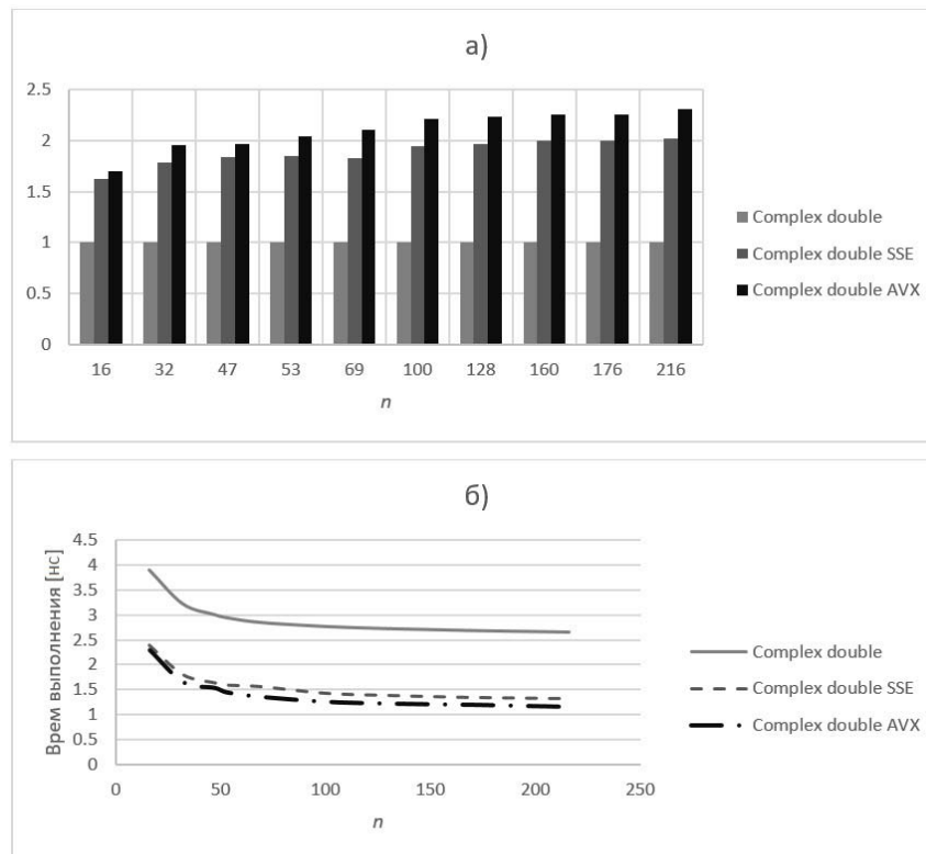
Рис. 12. Гистограмма (а) и скорость выполнения одной итерации (б) корреляционной свертки для различного n для чисел типа complex double
