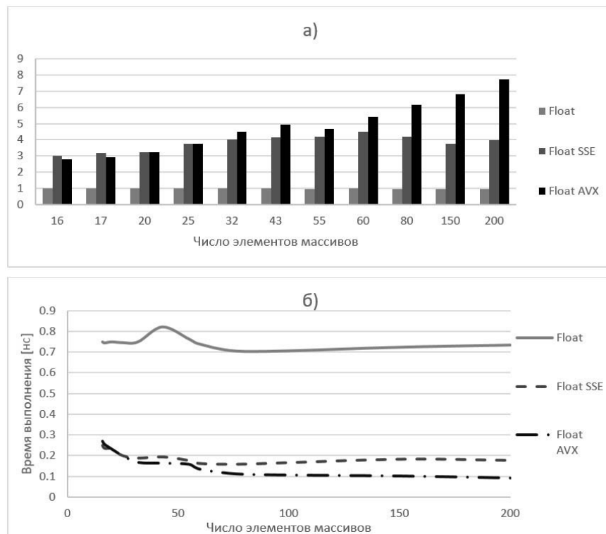
Рис. 1. Гистограмма (а) и скорость выполнения одной итерации (б) скалярного произведения для различного числа элементов в массивах для чисел типа float
