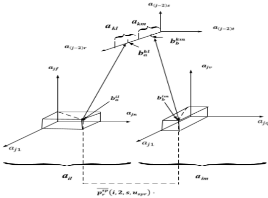
Рис.7. Геометрическая интерпретация экземпляра предметной зависимости 1-рода 2-го типа, где b_b^{km} – точка во фрагменте a_{km} оси a_{(j-2)r} , b_a^{kl} – точка во фрагменте a_{kl} оси a_{(j-2)r} , b_a^{il} – точка в пространстве a_{il} , b_b^{im} – точка в пространстве a_{im} [24]
