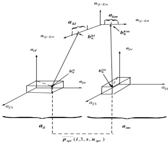
Рис.8. Геометрическая интерпретация экземпляров предметной зависимости 1-рода 3-го типа, где b_b^{km} – точка во фрагменте a_{km} оси a_{(j-2)t} , b_a^{kl} – точка во фрагменте a_{kl} оси a_{(j-2)t} , b_a^{il} – точка в пространстве a_{il} , b_b^{im} – точка в пространстве a_{im} [24]
