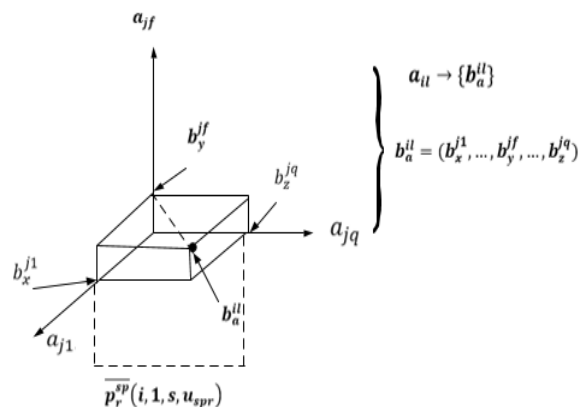
Рис.6. Геометрическая интерпретация экземпляров предметной зависимости 1-рода 1-го типа: a_{il} – пространство с осями a_{j1}, \dots, a_{jq}, \dots, a_{jf} , b_a^{il} – точка в пространстве a_{il} [24]
