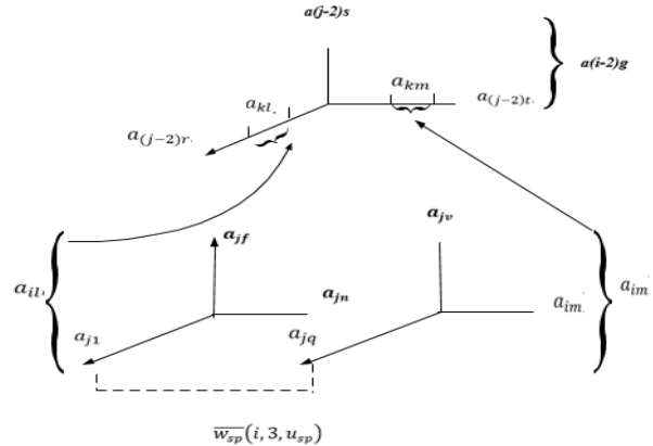
Рис.5. Геометрическая интерпретация предметной зависимости 1-го рода 3-го типа, где a_{il}, a_{im} – определяют абстрактные пространства, a_{j1}, \dots, a_{jq}, a_{jm}, a_{(j-2)r}, a_{(j-2)t} – определяют оси пространств разного уровня семантической сложности, a_{kl}, a_{km} – определяют фрагменты шкал на разных осях [24,25]
